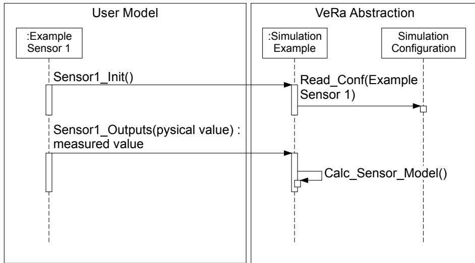
Abbildung 4.10: Sensoraufruf im Anwendungsfall Simulation dargestellt im Sequenzdiagramm
