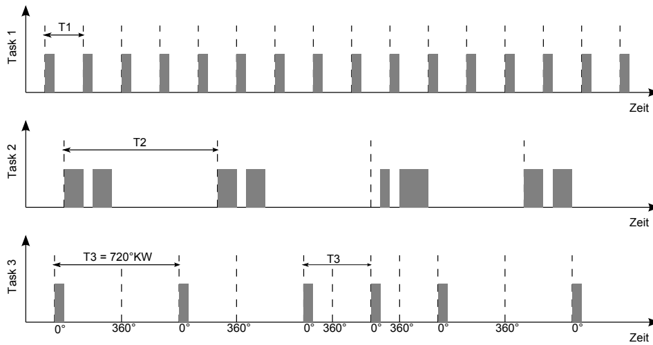
Abbildung 4.13: Beispiel eines Taskmodells, Task 1 ist zeitbasiert mit kleiner Periodendauer (T1), Task 2 ist zeitbasiert mit großer Periodendauer (T2), Task 3 ist winkelbasiert mit einer Periodendauer (T3)
