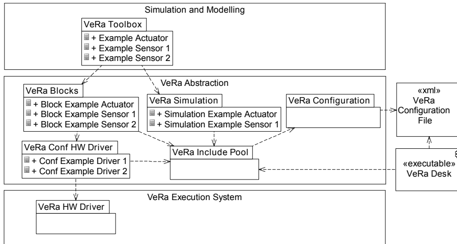
Abbildung 4.7: Klassendiagramm der VeRa Abstraktionsschicht
