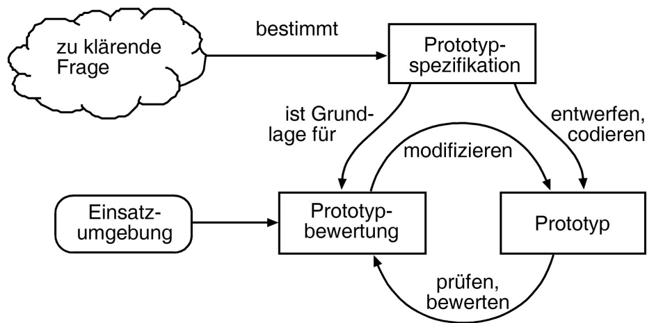
Abbildung 2.5: Allgemeine Vorgehensweise beim Prototyping [41]
