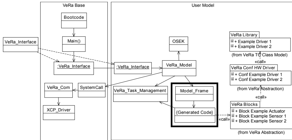
Abbildung 6.16: Klassendiagramm des VeRa Ausführungssystems. Das Aufrufmodul sowie der mit Targetlink generierte Code sind schwarz umrandet.
