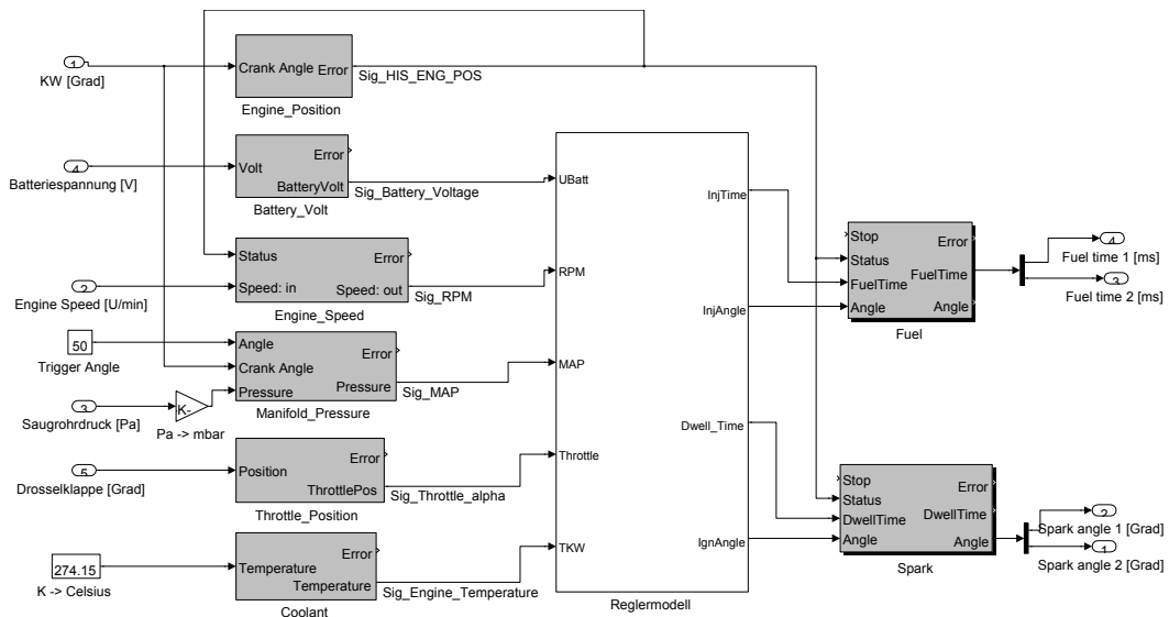
Abbildung 6.3: Das Modell mit Verwendung der Abstraktionsschicht [61]
