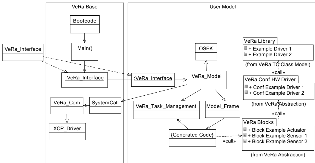
Abbildung 4.14: Das VeRa Ausführungssystem im Klassendiagramm
