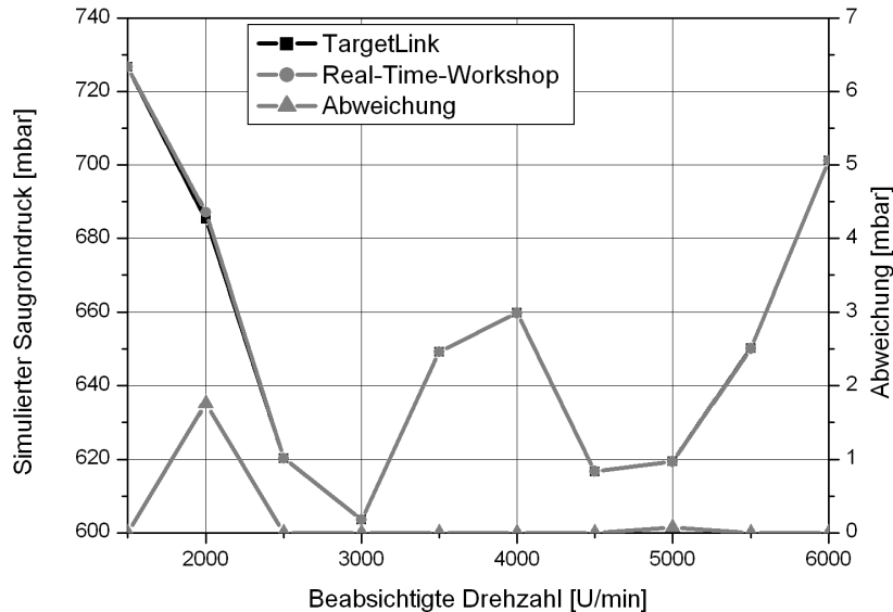
Abbildung 6.17: Vergleich der Targetlink und der Simulink Simulationsergebnisse bei einem effektiven Mitteldruck von 4bar.
