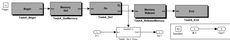
Abbildung 6.9: Berechnung im Subsystem aller Tasks
