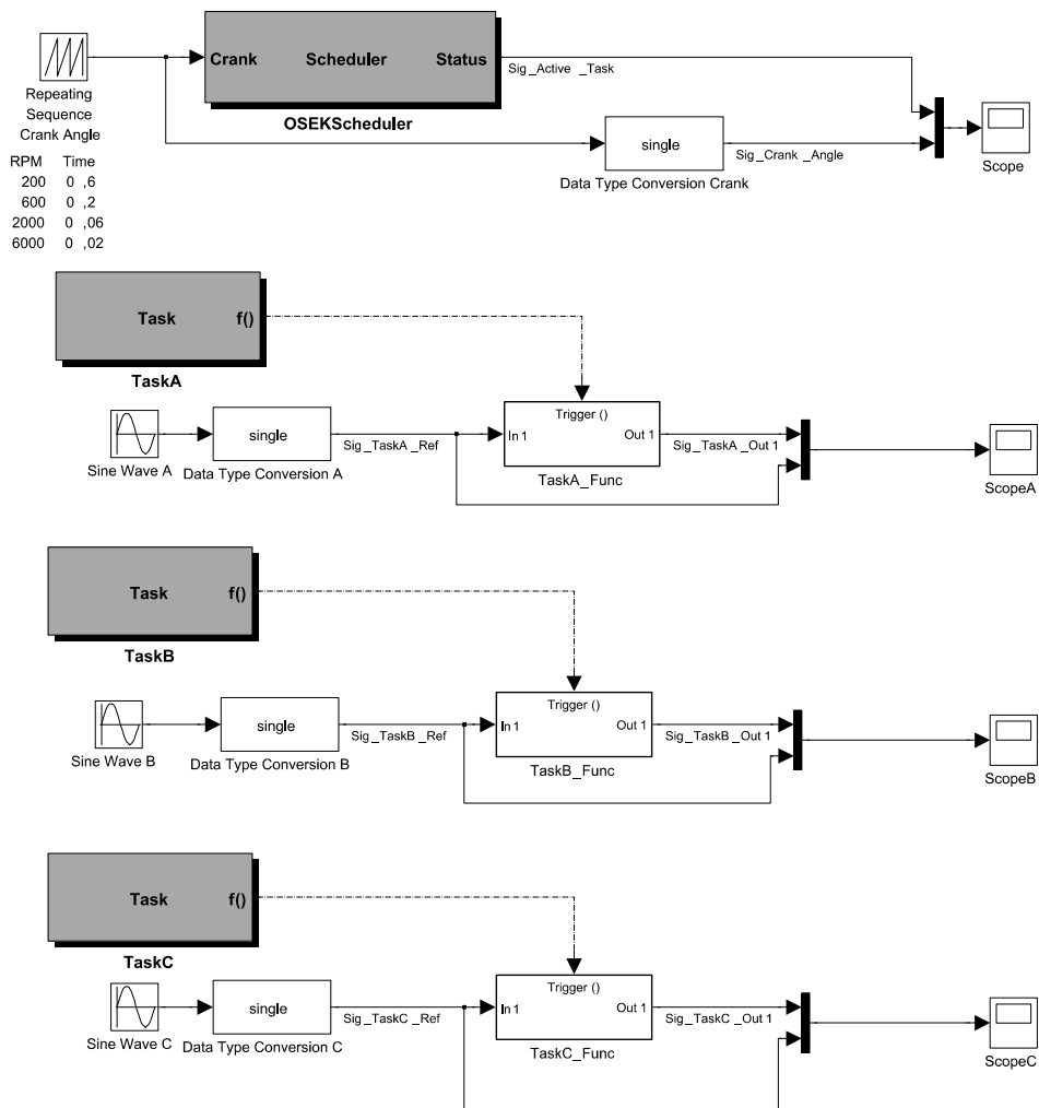
Abbildung 6.8: Versuchsmodell bestehend aus drei Tasks
