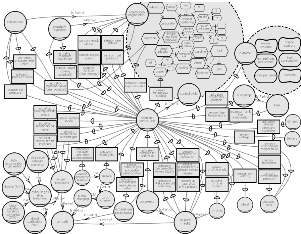
Abbildung 5.2: Generisches Domänenmodell für Motorsteuerungssysteme [56]
