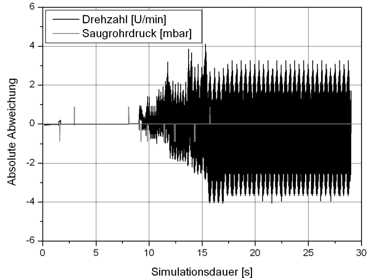
Abbildung 6.18: Zeitliche Entwicklung und Stabilisierung des absoluten Abweichung zwischen dem Targetlink und dem Simulink Modell angegeben für die Größen Drehzahl und Saugrohrdruck
