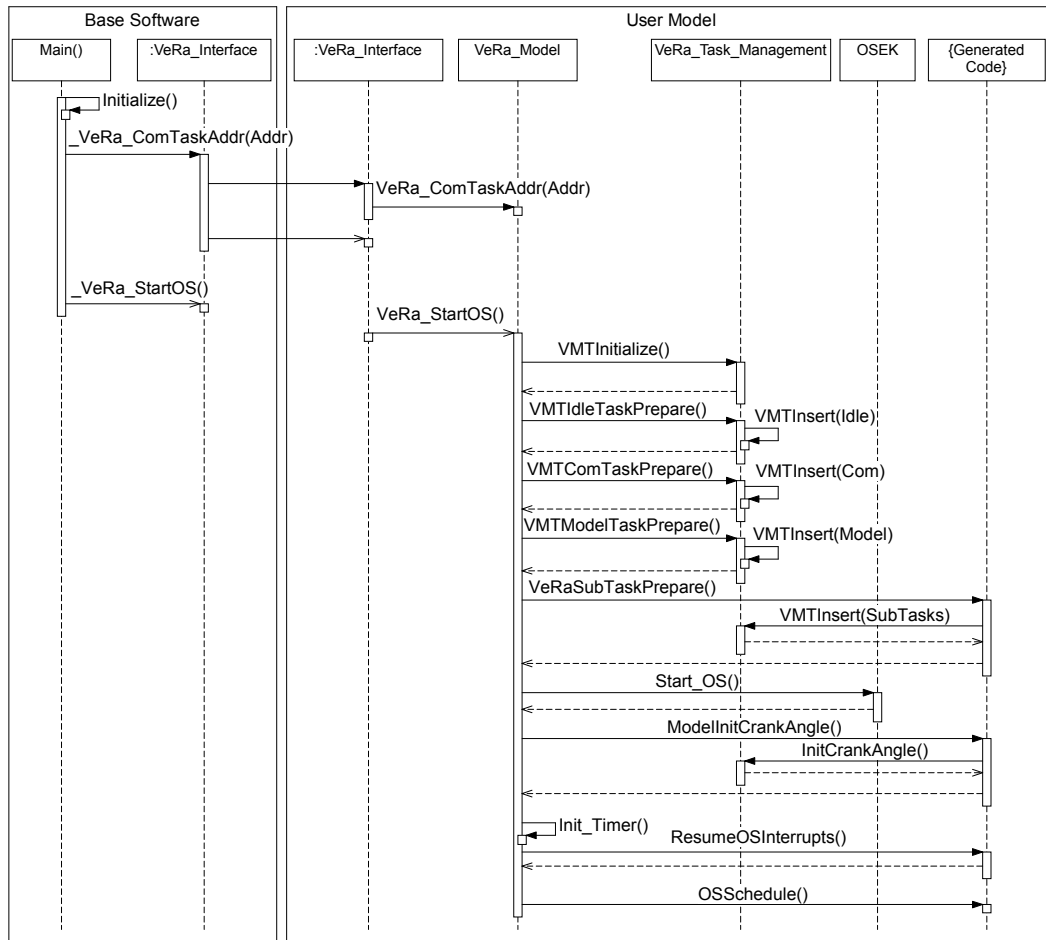
Abbildung 4.15: Startsequenz des VeRa Ausführungssystems
