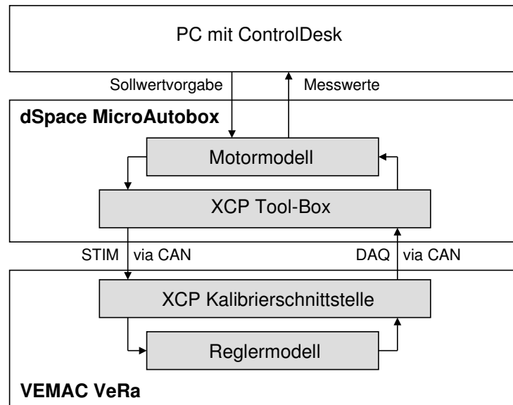
Abbildung 6.13: Schematischer Versuchsaufbau [21]
