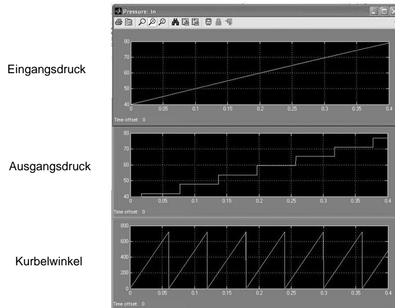
Abbildung 6.5: Testergebnisse des Block Manifold Pressure [61]
