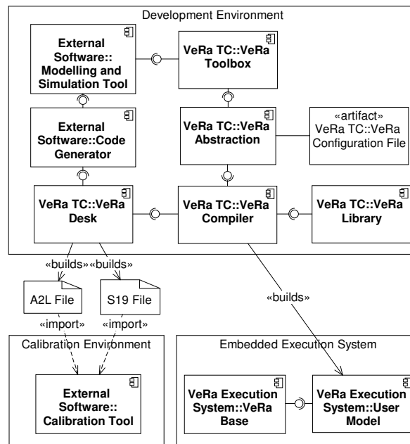
Abbildung 4.6: Das VeRa System im Komponentendiagramm
