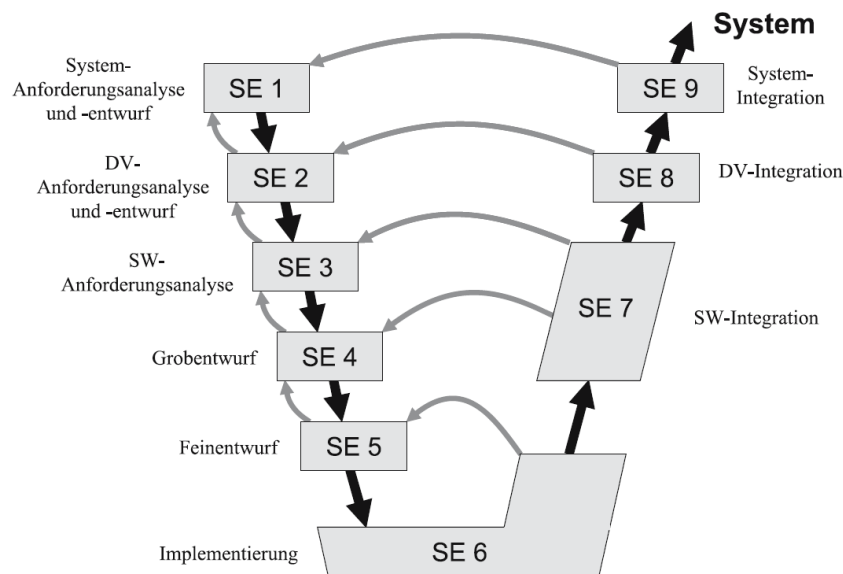
Abbildung 2.7: V-Modell 97: Tätigkeiten zur Systemerstellung [52]
