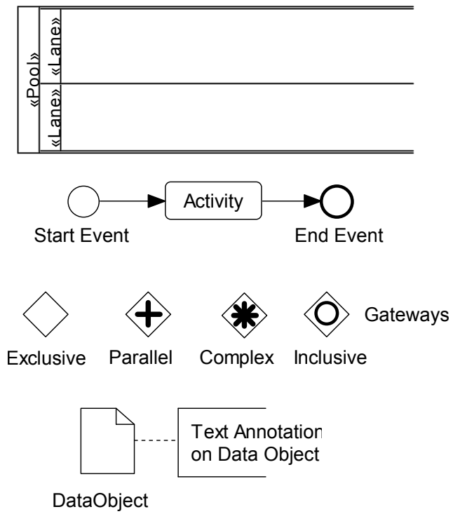
Abbildung 2.11: Einige Basis-Notationselemente der BPMN
