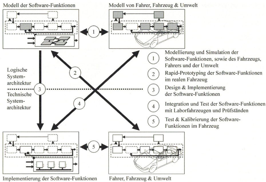
Abbildung 2.2: Modellbasierte Entwicklung aus [54]
