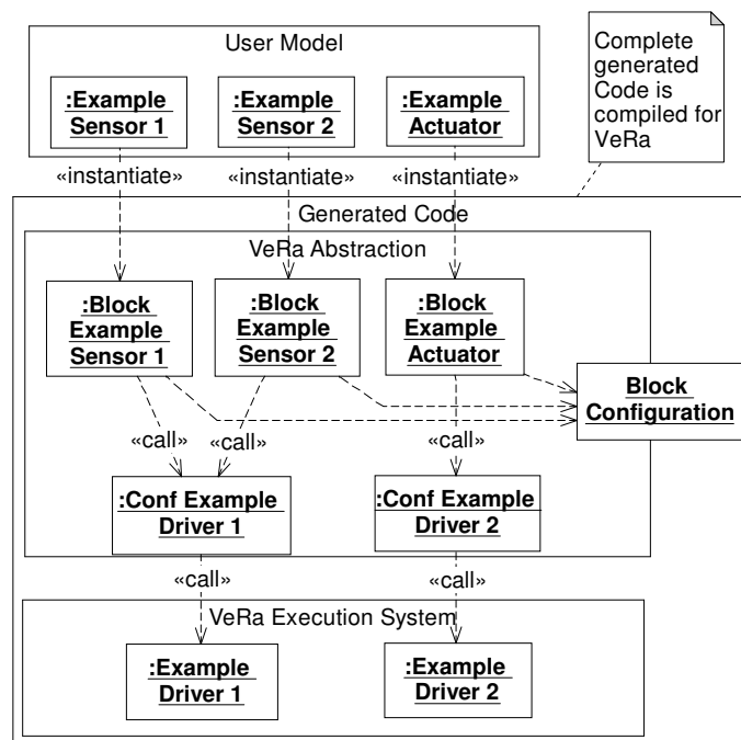
Abbildung 4.11: Objektdiagramm für den Anwendungsfall Code Generierung
