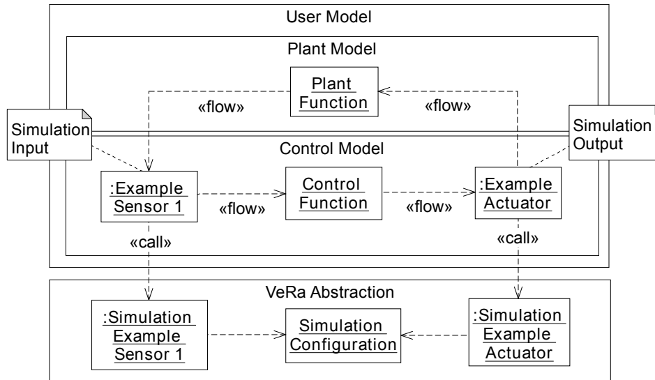
Abbildung 4.9: Objektdiagramm für den Anwendungsfall Simulation
