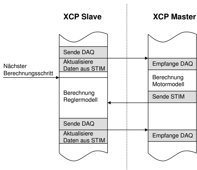
Abbildung 6.12: HIL-System mit XCP-Verbindung [21]
