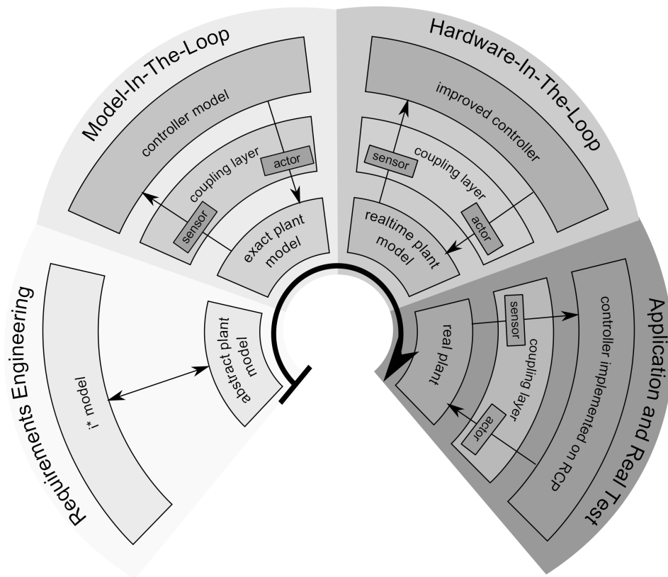
Abbildung 2.1: ZAMOMO-Entwicklungsprozess für softwareintensive Regelungssysteme [51]
