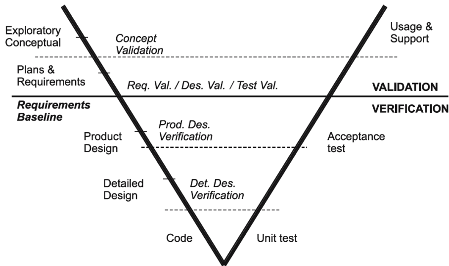
Abbildung 2.6: Das V-Modell nach Boehm [9]
