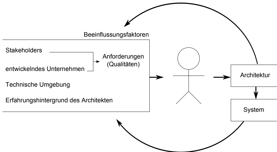
Abbildung 2.4: Architecture Business Cycle nach [6]
