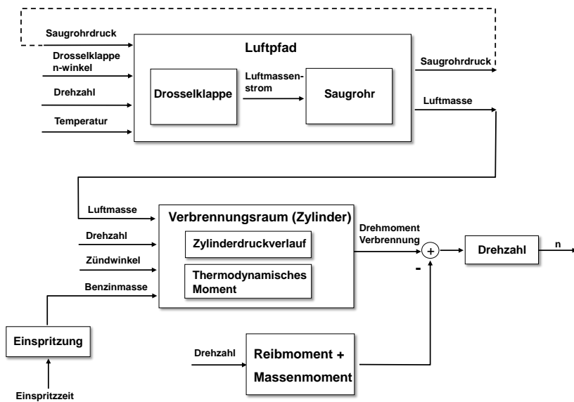
Abbildung 6.2: Modulare Modellstruktur [61]
