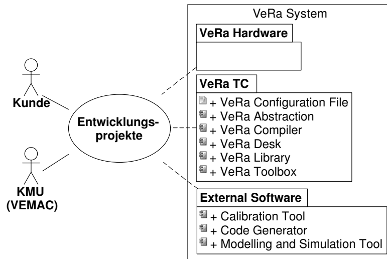
Abbildung 4.1: Grundlegendes Use Case Diagramm
